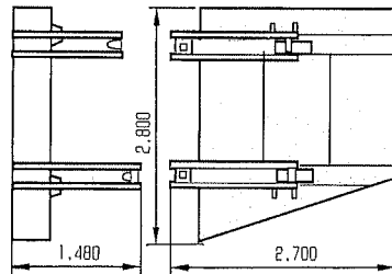
●カウンタウイト架台 質量：14.0ton×2
