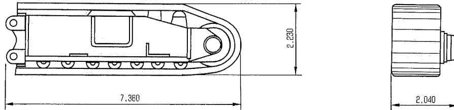
●クローラ前 質量：32.4ton×2 (シューなし20.5ton×2)
