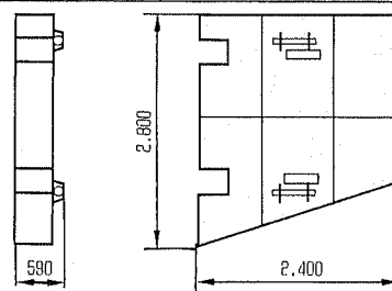
●No1カウンタウイト 質量：14.0ton×2
