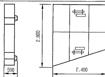
●No2カウンタウイト 質量：14.0ton×2
